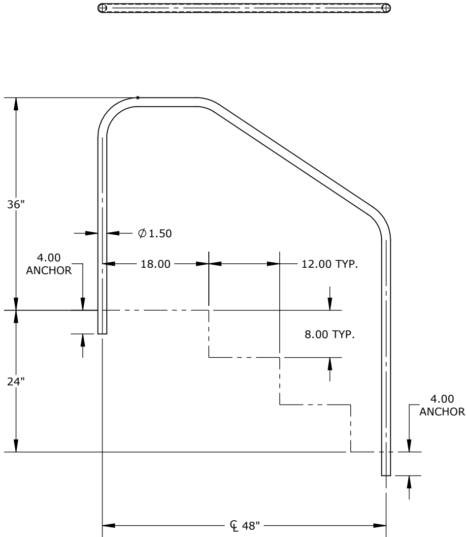
TRUPRO - 3-BEND STAIR RAIL - 48.00" LONG X 1.50" OD X .120 WALL - 316LSS
