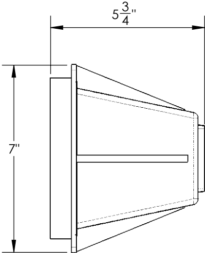
SCALE 1 : 3.5
