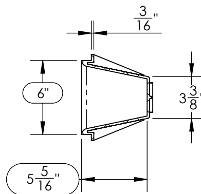
SECTION B-B SCALE 1 : 8
